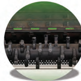
Rotor de concasseur en carbure دوار كسارة الكريبد
